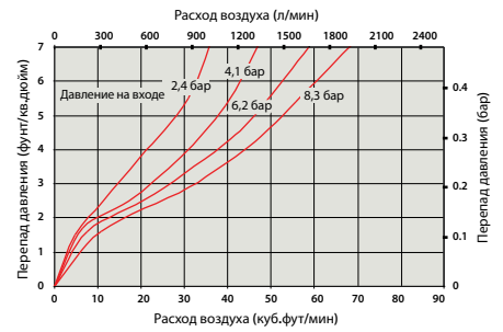
Лубрикатер 1/4" - перепад давления
