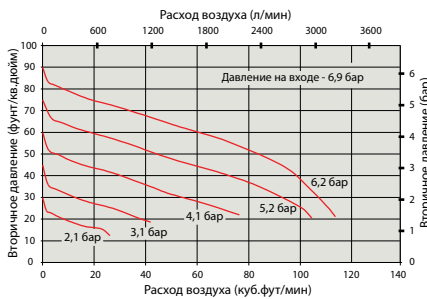
Ф/Р+Л 3/8" - перепад давления
