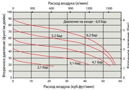
Ф/Р+Л 1/4" - перепад давления
