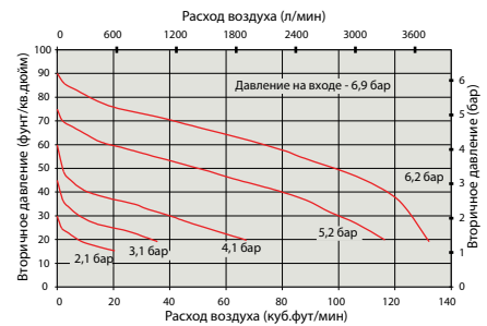
Ф+Р+Л 3/8" - перепад давления
