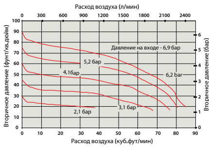
Регулятор 1/4" - перепад давления
