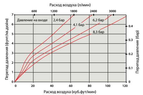
Лубрикатер 3/8" - перепад давления
