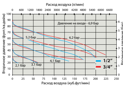
Ф/Р+Л 1/2" и 3/4" - перепад давления
