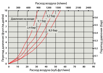
Фильтр 1/4" - перепад давления
