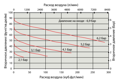
Ф+Р+Л 1" - перепад давления
