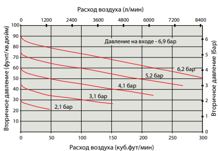
Фильтр-регулятор 1" - перепад давления
