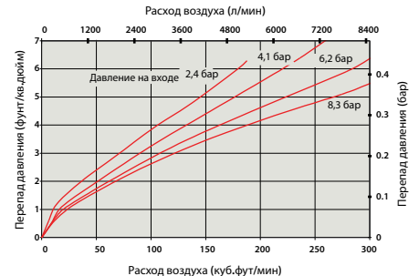
Лубрикатер 1" - перепад давления
