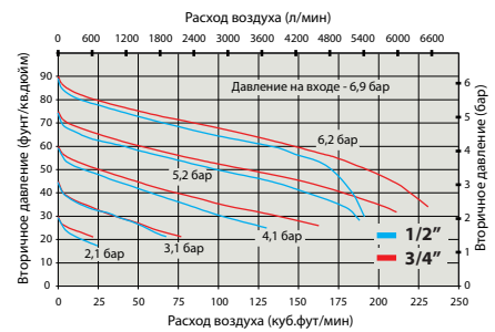
Ф+Р+Л 1/2" и 3/4" - перепад давления
