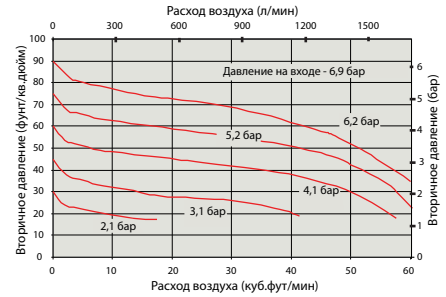
Ф+Р+Л 1/4" - перепад давления
