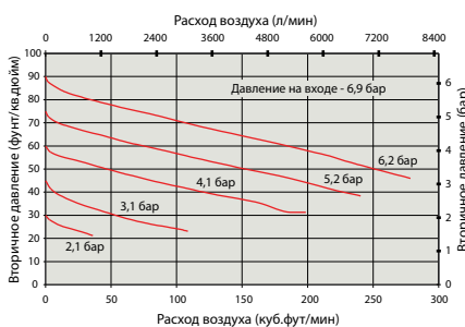
Ф/Р+Л 1" - перепад давления
